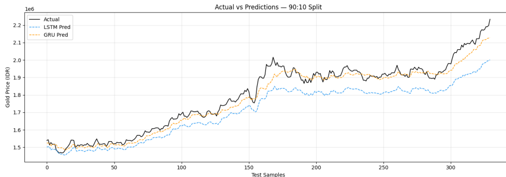
Gambar 8. Line Chart Actual vs Prediction GRU dan LSTM (Split 90:10)
