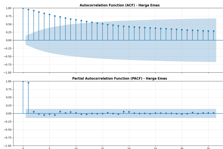
Gambar 6. Analisis ACF dan PACF
