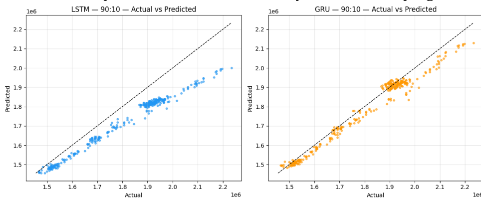
Gambar 9. Scatter Plot Actual vs Predicted - GRU dan LSTM (Split 90:10)
