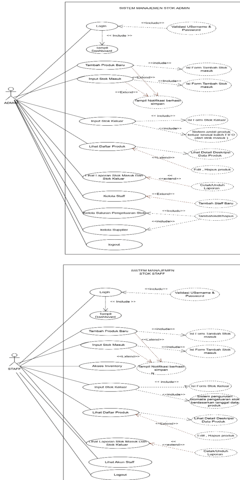
Gambar 3. Use Case Diagram Admin dan Staff
