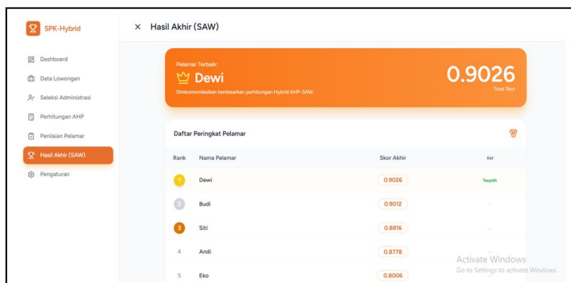
Gambar 10. Perangkingan (SAW)
