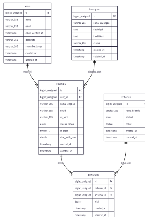
Gambar 6. Desain database
